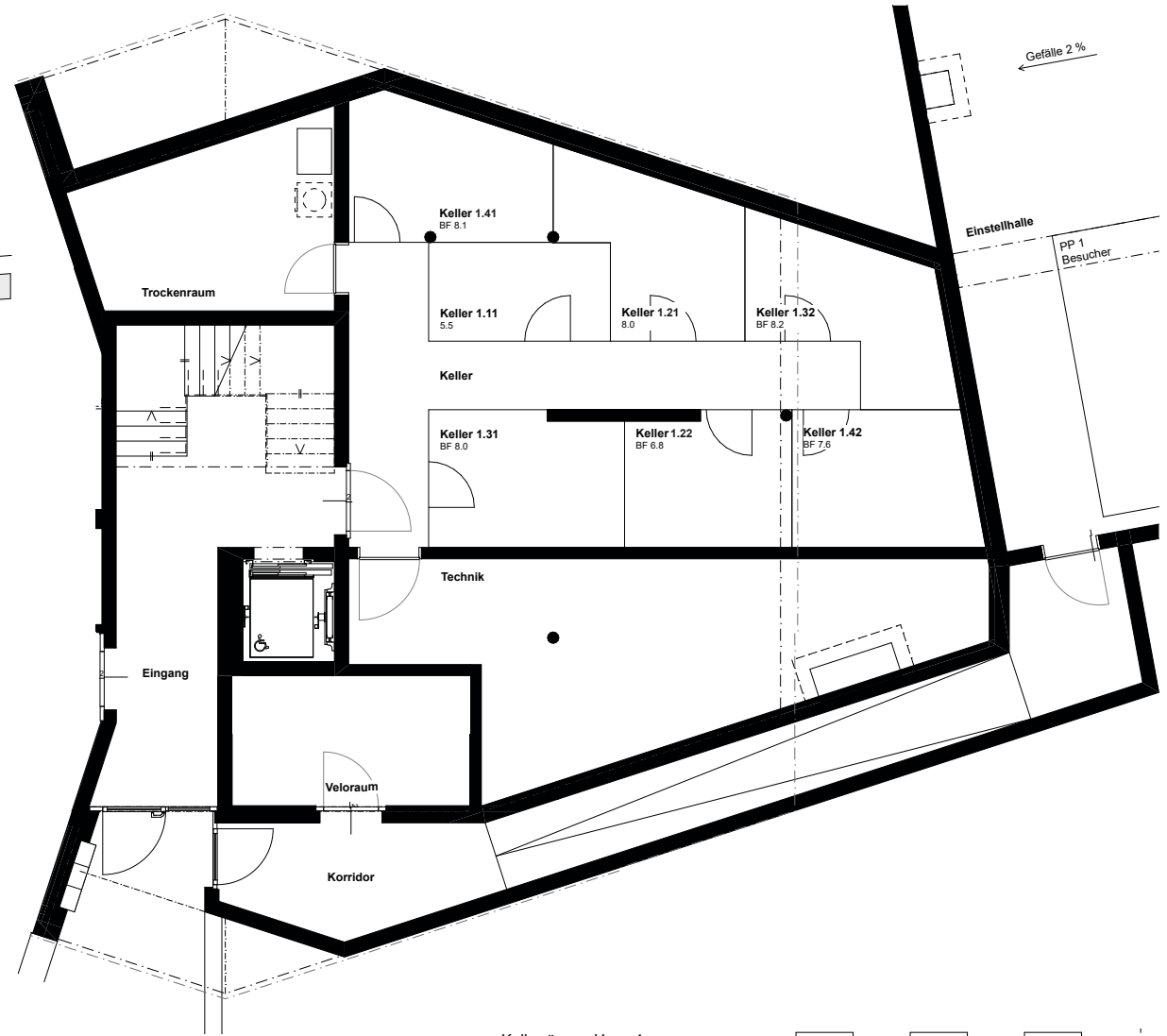
Kellerräume Haus 1 0 1 2 3 4 5m M 1:100
